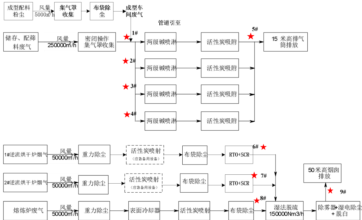
图 7.1-2 有组织废气检测布点示意图
