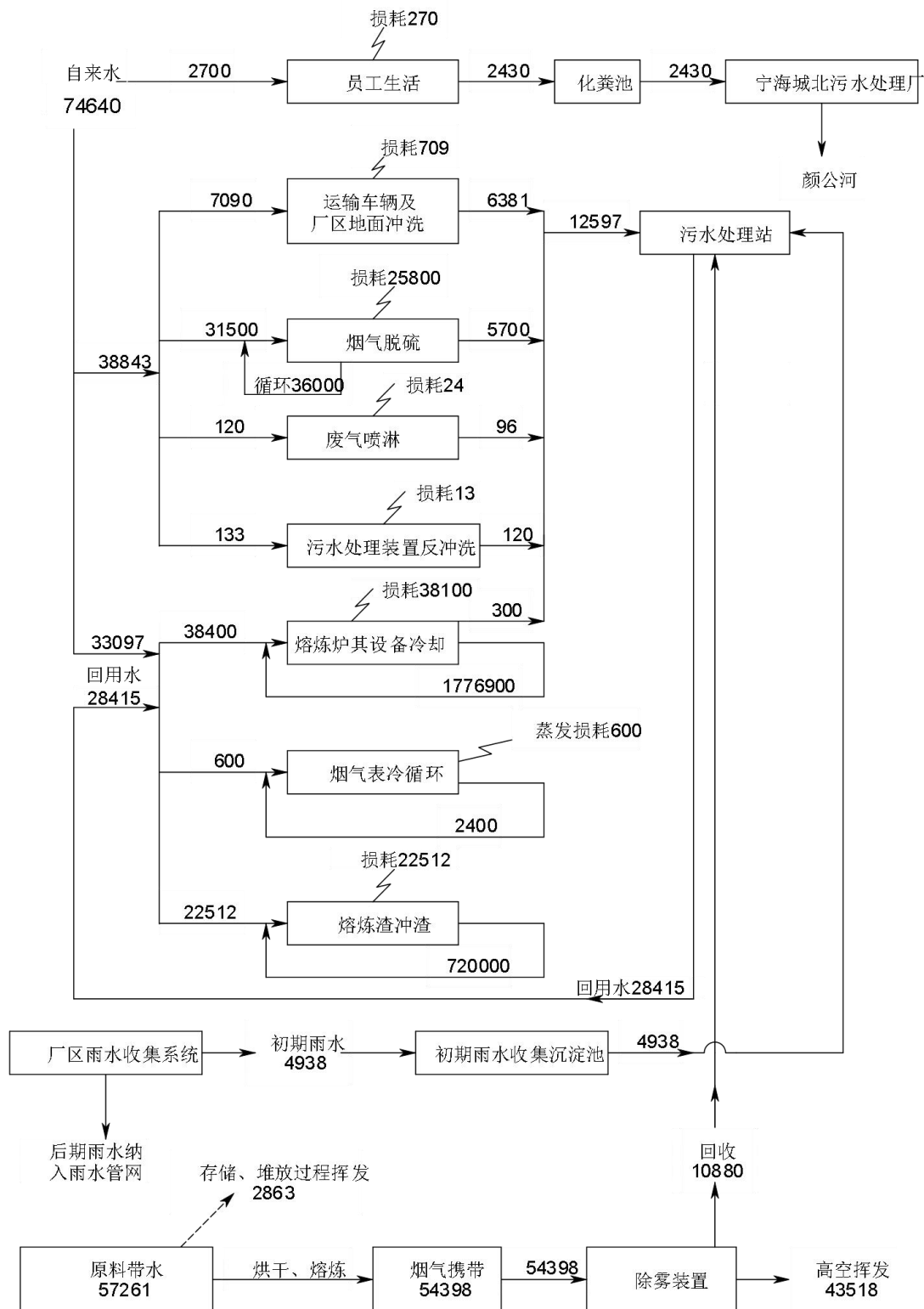
图 3.3-1 本项目实际运行期间水平平衡图
