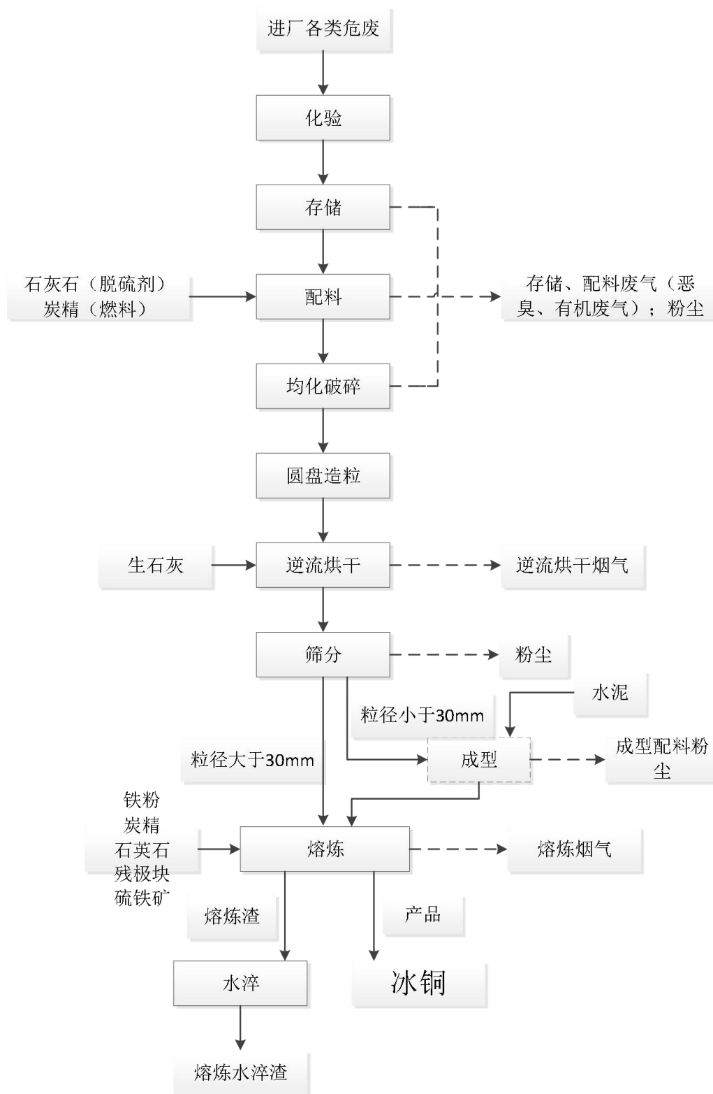
图 3.4-2 实际生产工艺
