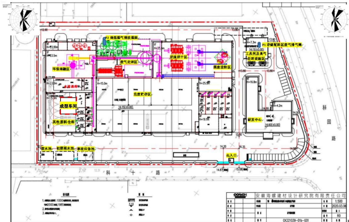
图 3.1-3 实际建设总平面布置图
