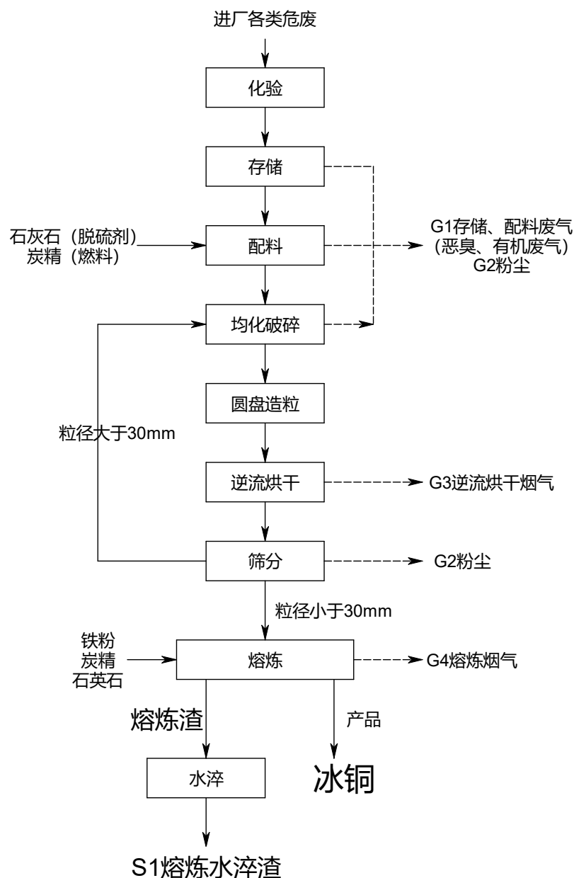
图 3.4-1 环评中的生产工艺
