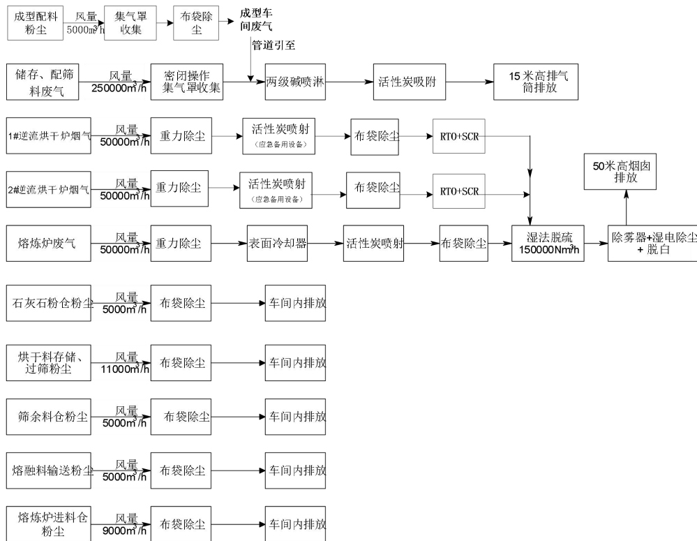
图 4.1-1 项目实际废气处理措施情况图
