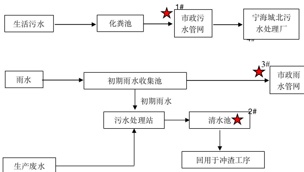
图 7.1-1 废水检测布点示意图
