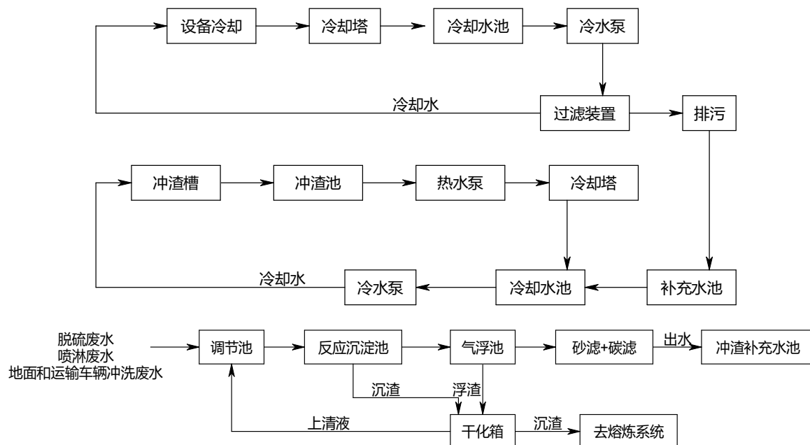
图 4.1-3 项目生产废水处理工艺流程图
